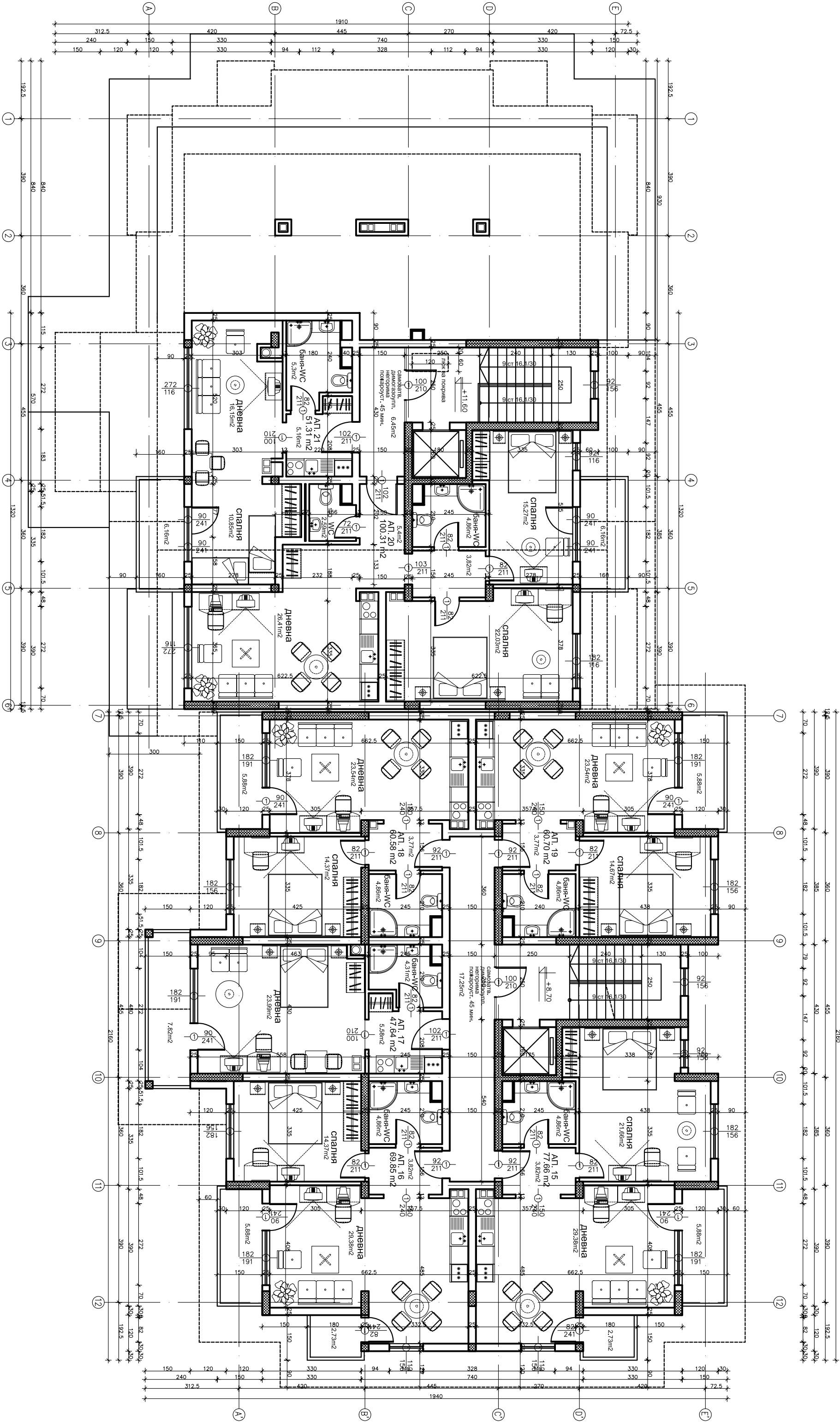
РАЗПРЕДЕЛЕНИЕ КОТА +1.60
