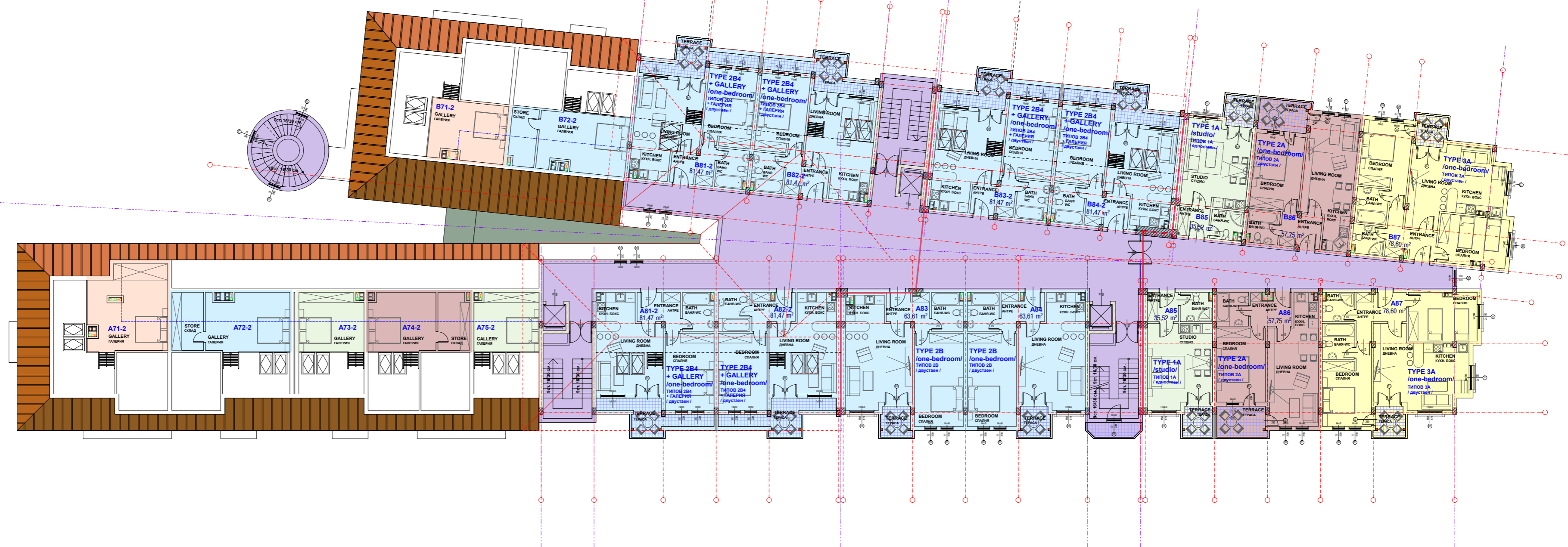
PLAN 8th STORY LEVEL +23,68 scale 1'200 РАЗПРЕДЕЛЕНИЕ ОСМИ ЭТАЖ КОТА +23,68 М 1'200
